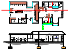
SECCIÓN LONGITUDINAL MUNICIPIO OFICINA LA DESCUBIERTA A LOCAL BIBLIOTECA MUNICIPAL
